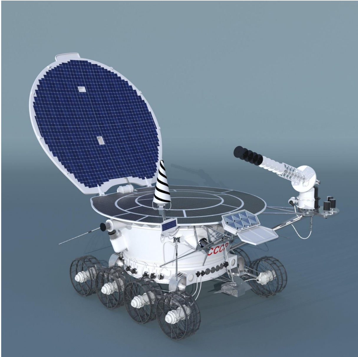
Łazik radziecki Łunoход 1 – model komputerowy (odtworzenie). Źródło: NASA
